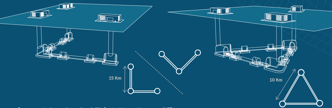
Rappresentazione schematica dell'infrastruttura sotterranea di ET e delle due possibili configurazioni, e la sua localizzazione in Sardegna Schematic representation of ET underground infrastructure and of the two possible configurations, and its location in Sardinia
